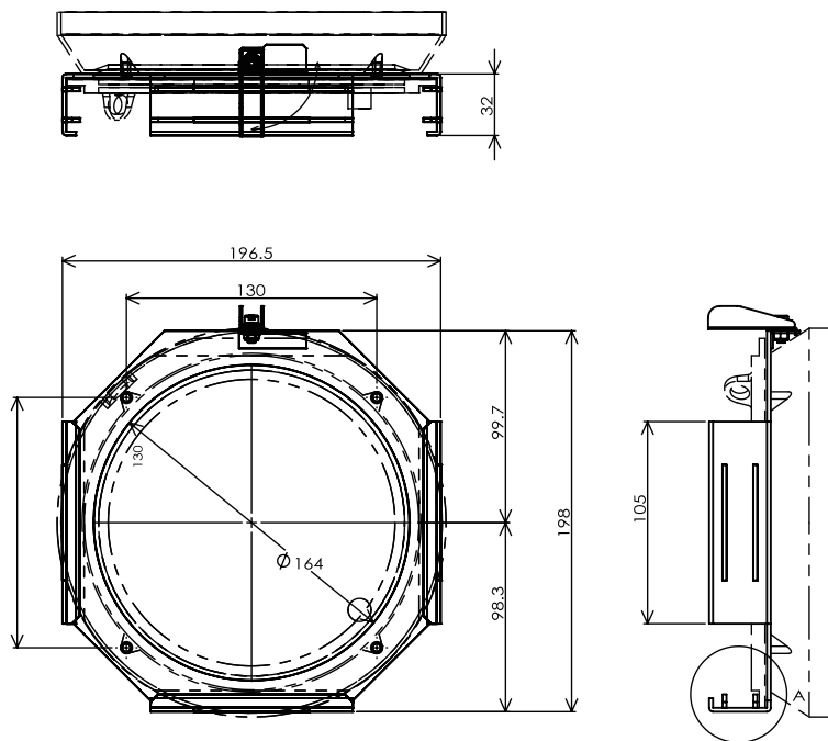
【LiZ-Frame寸法図】
